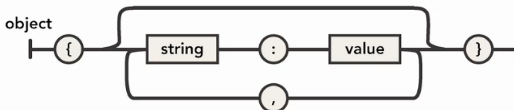
Abbildung 1: json.org
